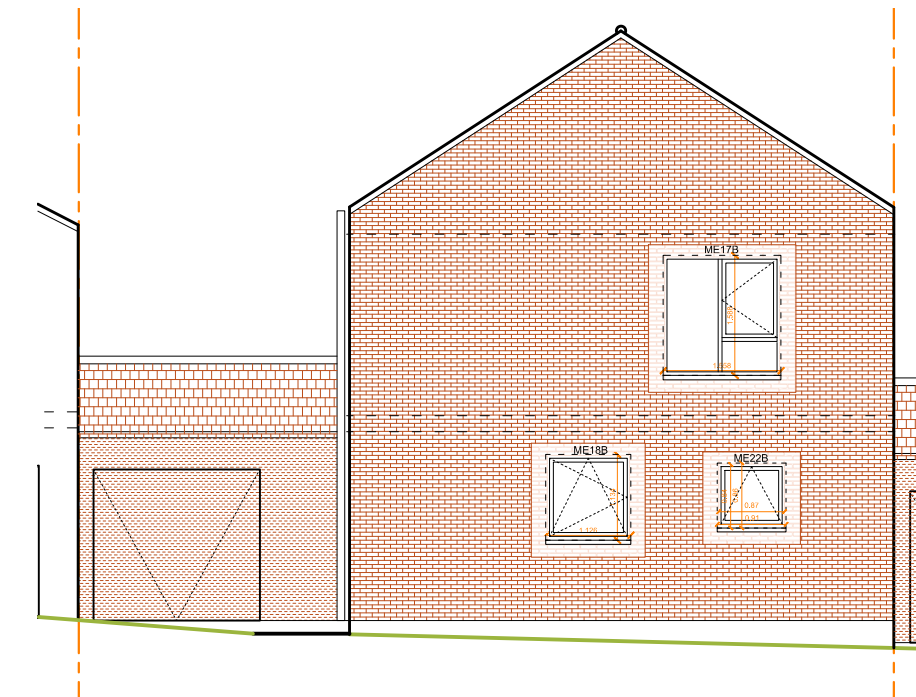
Façade nord
