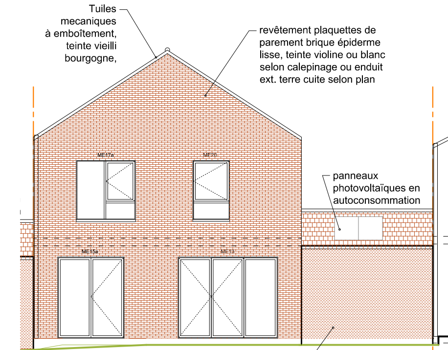
Façade sud
