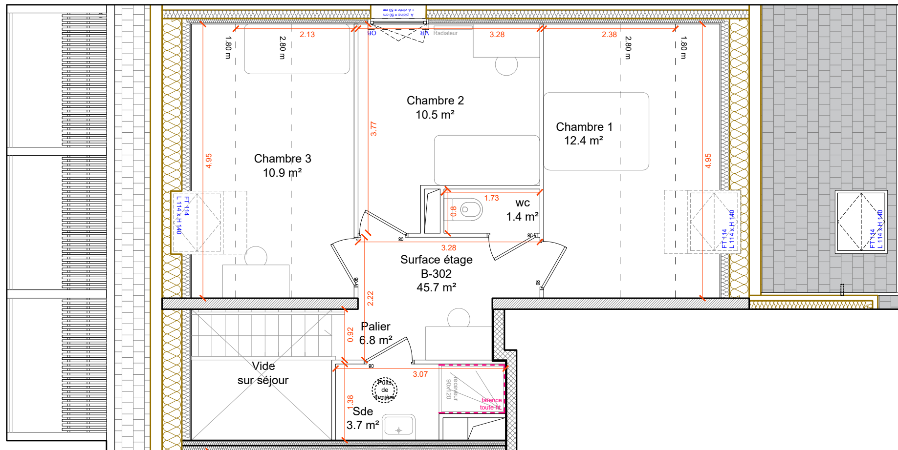
R+4 - Etage
